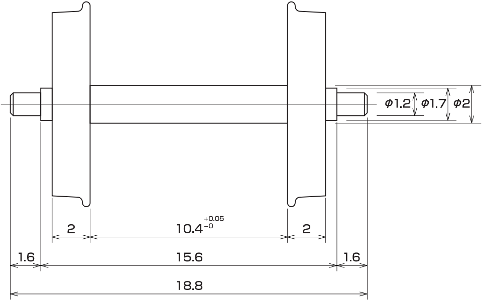
短軸プレーン車輪
