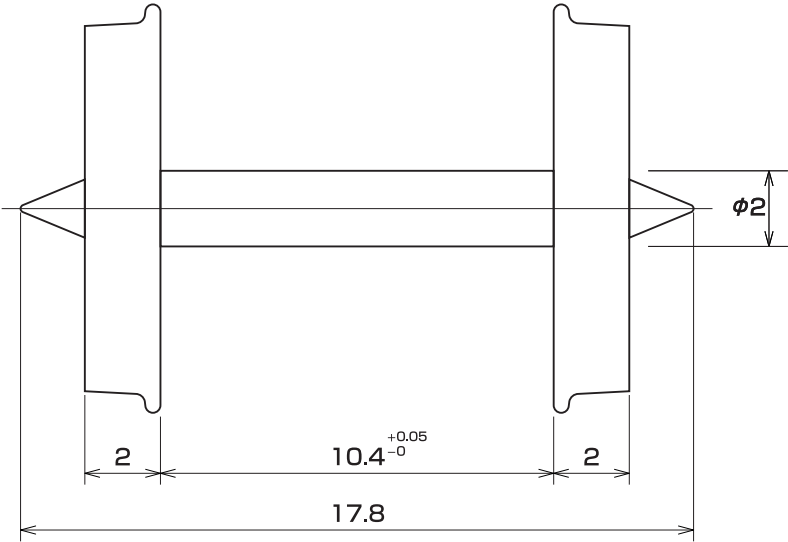
短軸ピボット車輪
