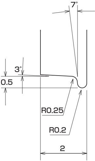
フランジ形状
