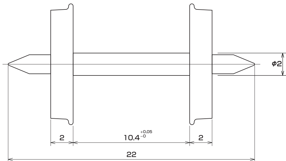
長軸ピボット車輪
