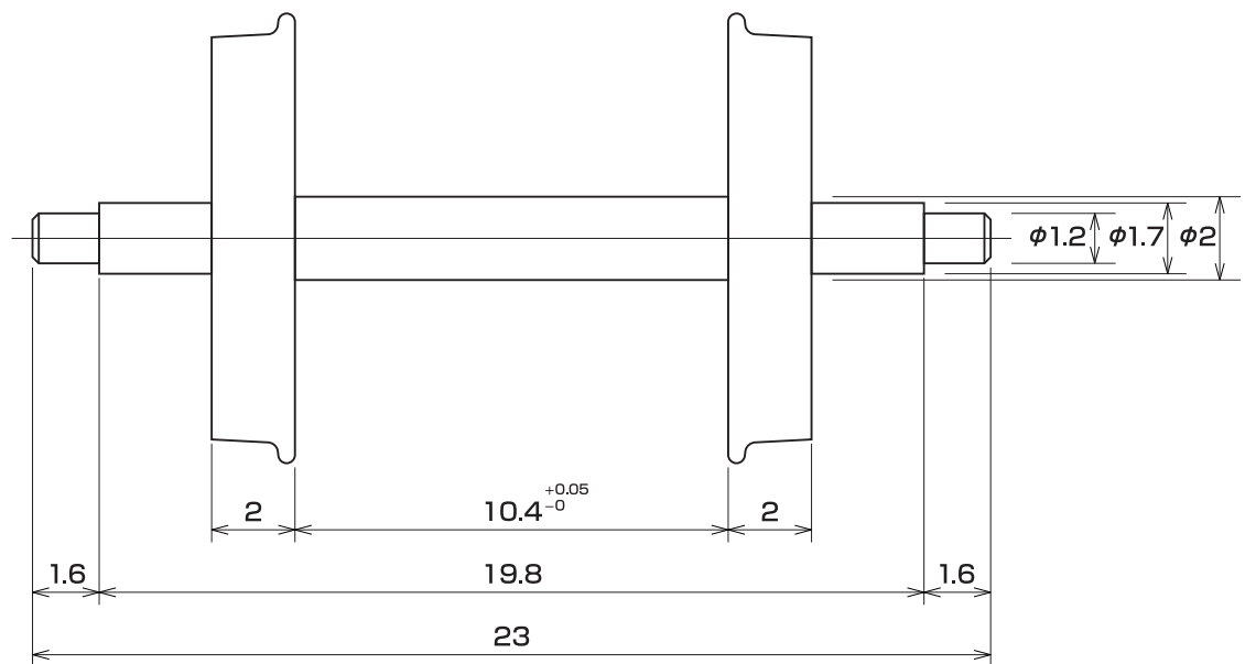
長軸プレーン車輪
